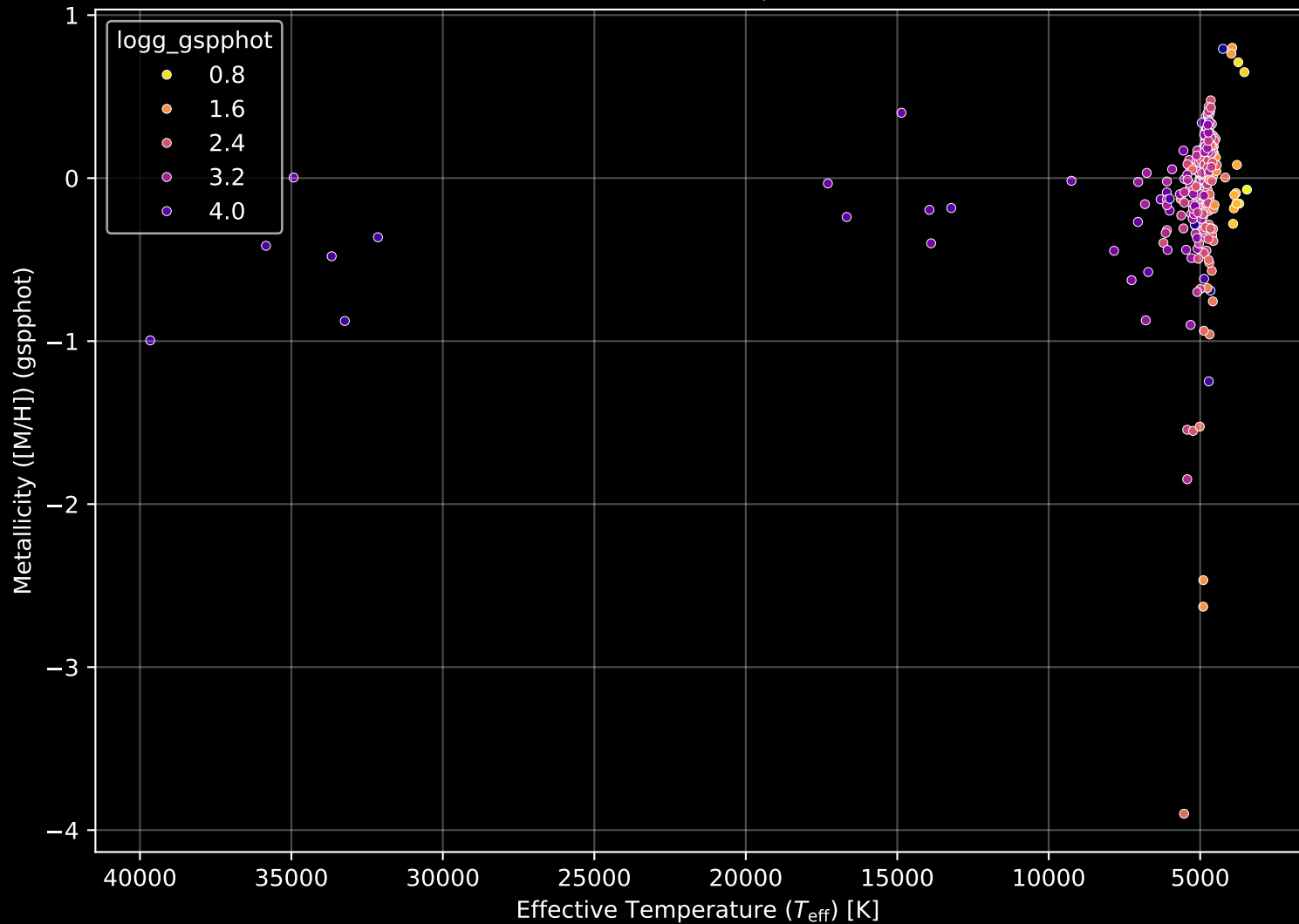
APOGEE DR17 Field: [350+04] Stellar Population Parameters (n= 343)
